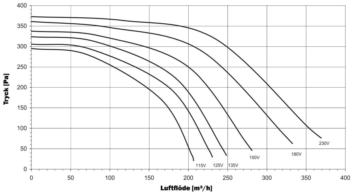
Tryck/Luftflöde diagram
