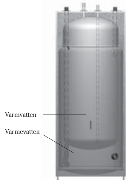
Dubbelmantlad varmvattenberedare
