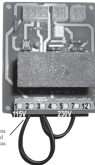
Styrkort
