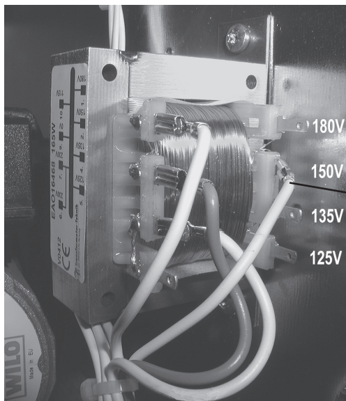
Fläkttransformator
