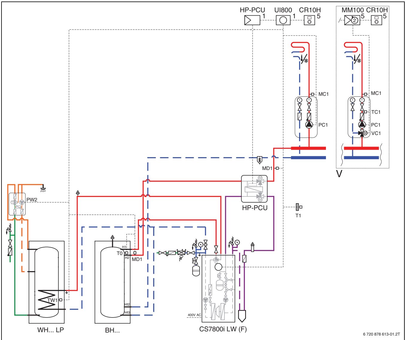
Bild 13 Bufferttank, parallell med kylstation
